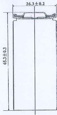
图 1 电芯外观尺寸
